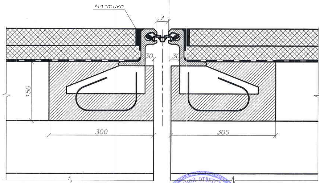
Конструкция деформационного шва СК-80
